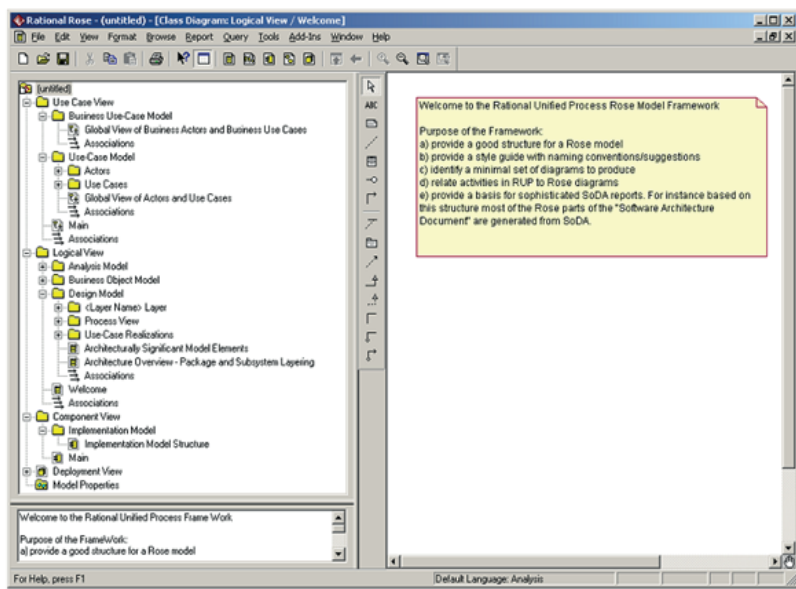
Рис. 4.1. Интерфейс среды Rose
