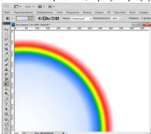
Рисунок 18 – Радуга Рассела
